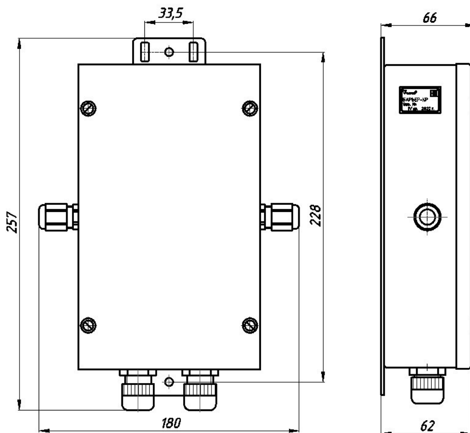
Рисунок 1 – Внешний вид коробки (стандартная комплектация)
